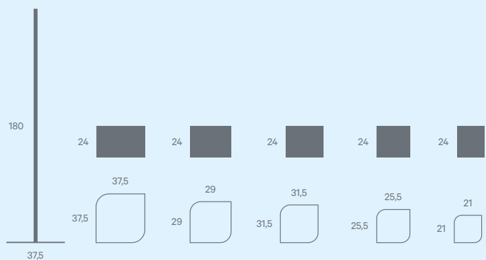
Bibliothèque modulaire | Modular bookshelf
