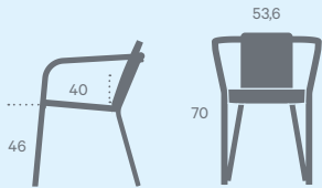
Fauteuil | Armchair (AL) 9 kg ☀️ 🚫
